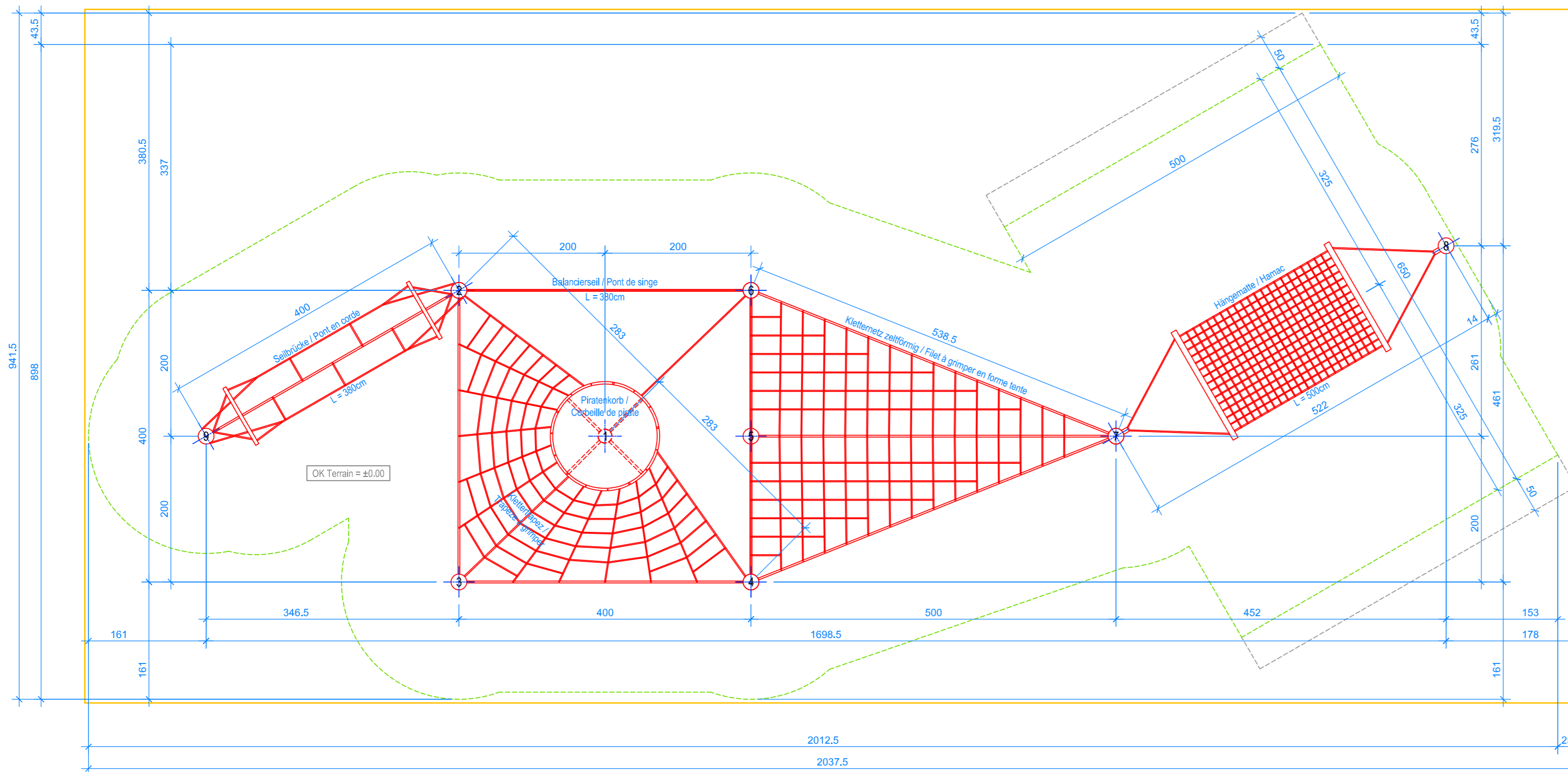
GRUNDRISS / PLAN 1:50
