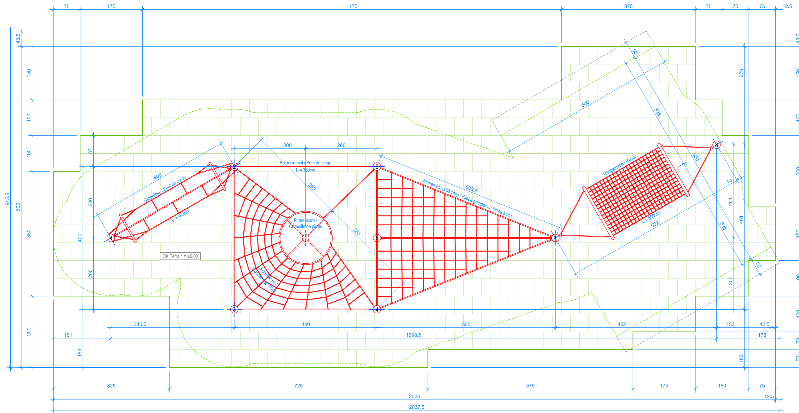
GRUNDRISS / PLAN 1:50
