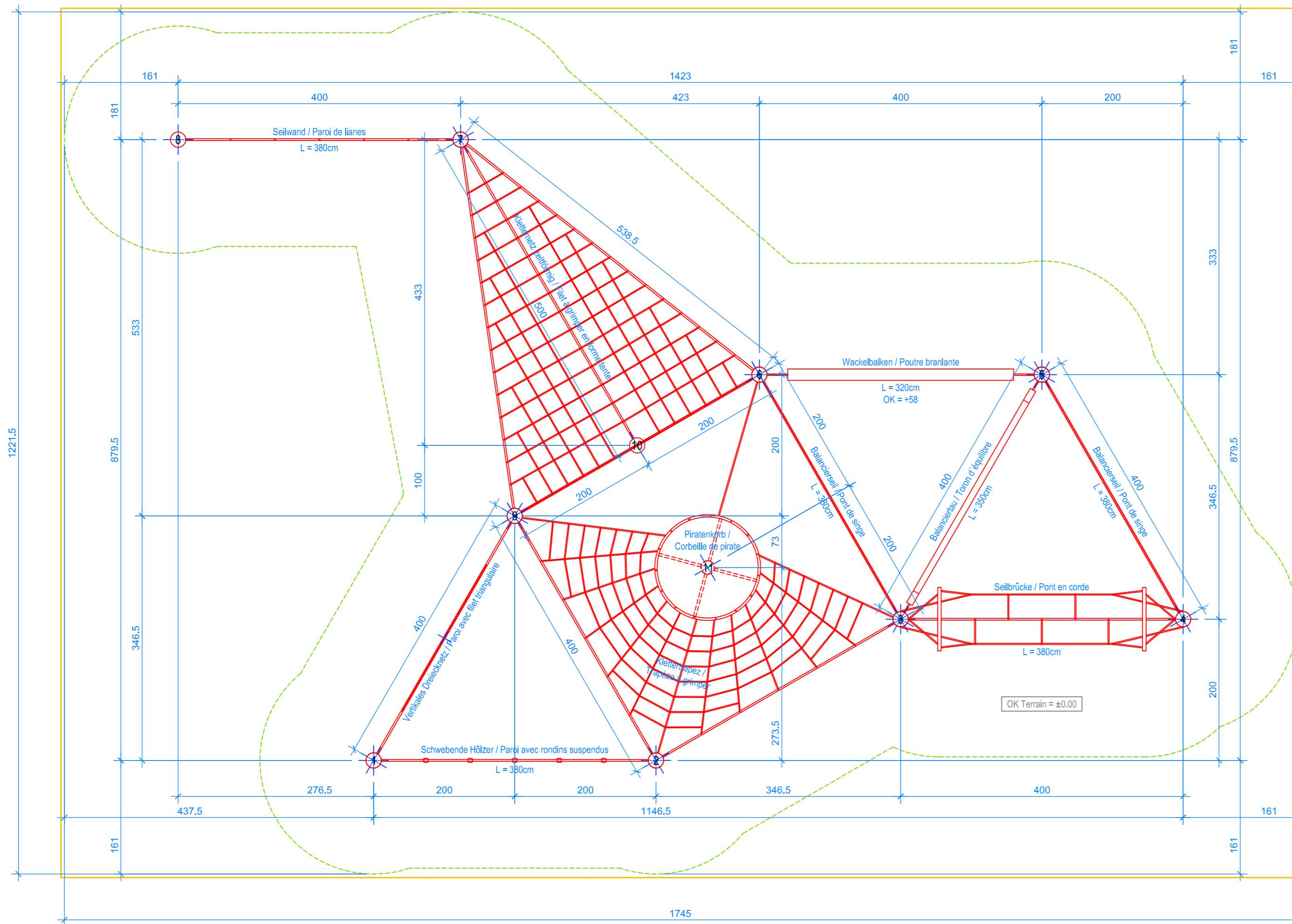
GRUNDRISS / PLAN 1:50
