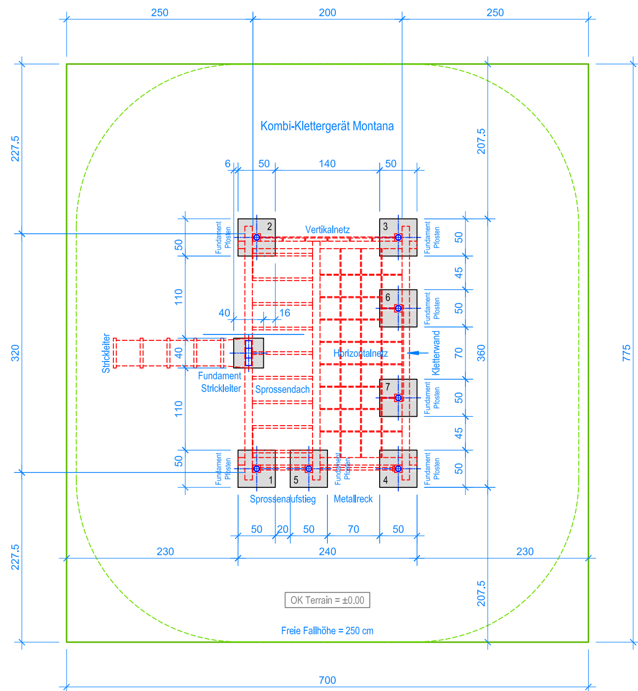
GRUNDRISS 1:50
