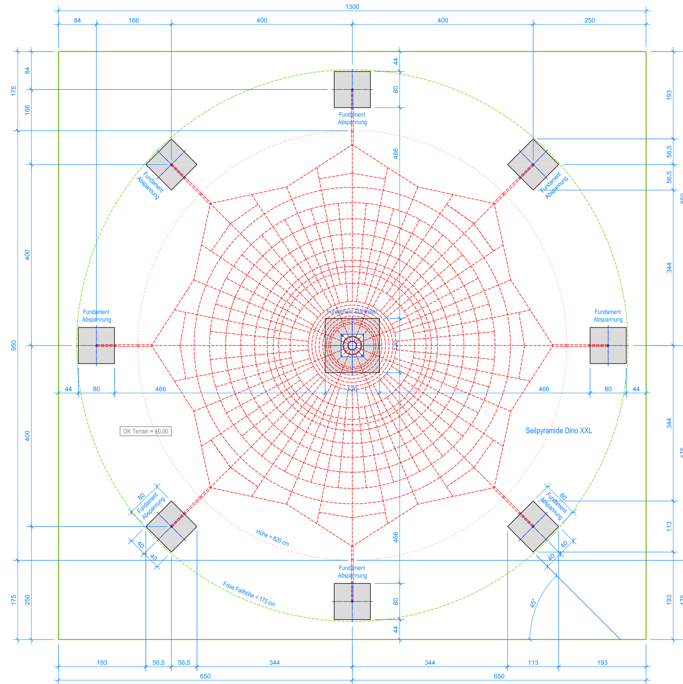
GRUNDRISS 1:50
