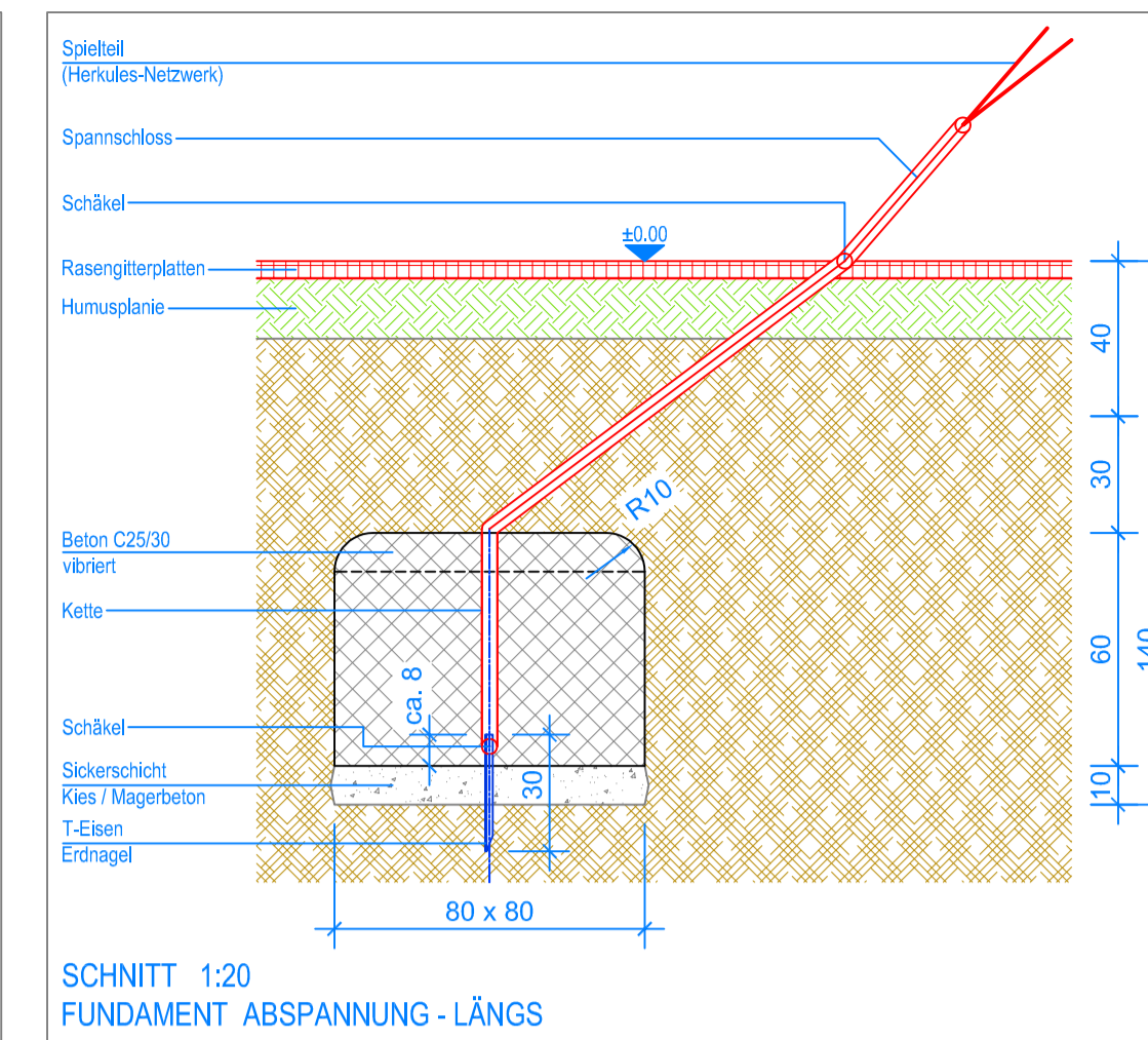
SCHNITT 1:20 FUNDAMENT ABSpannung - LÄNGS
