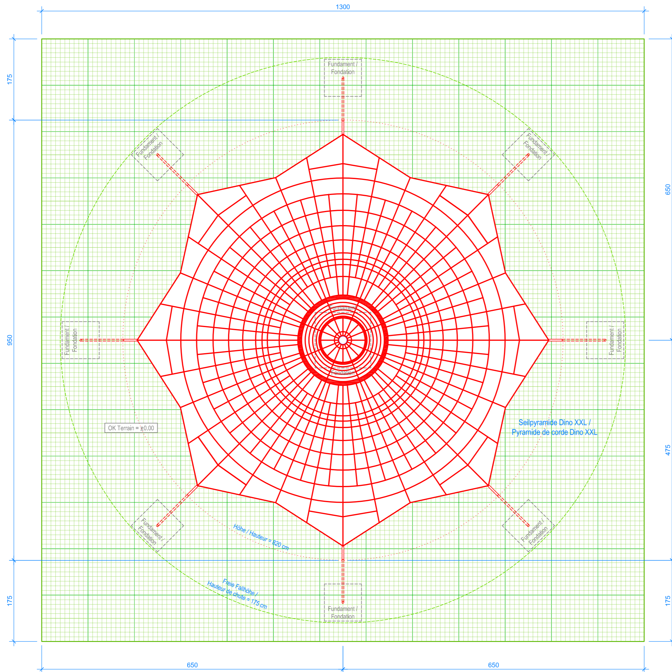
GRUNDRISS / PLAN 1:50
