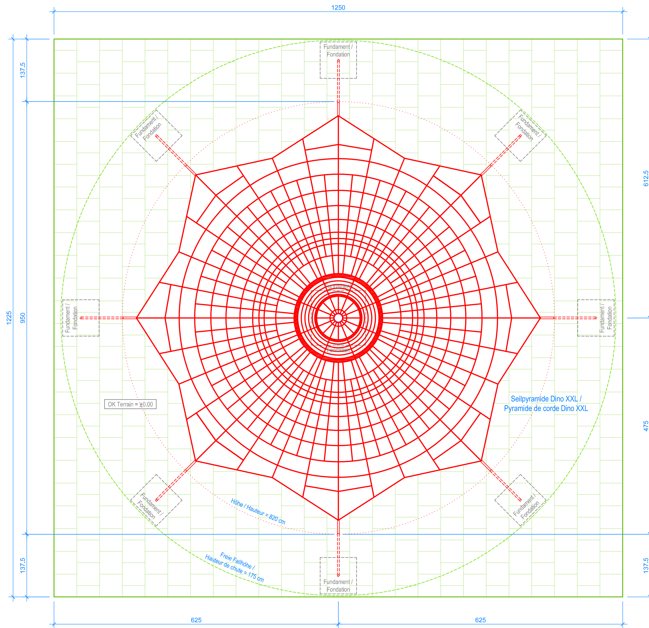
GRUNDRISS / PLAN 1:50
