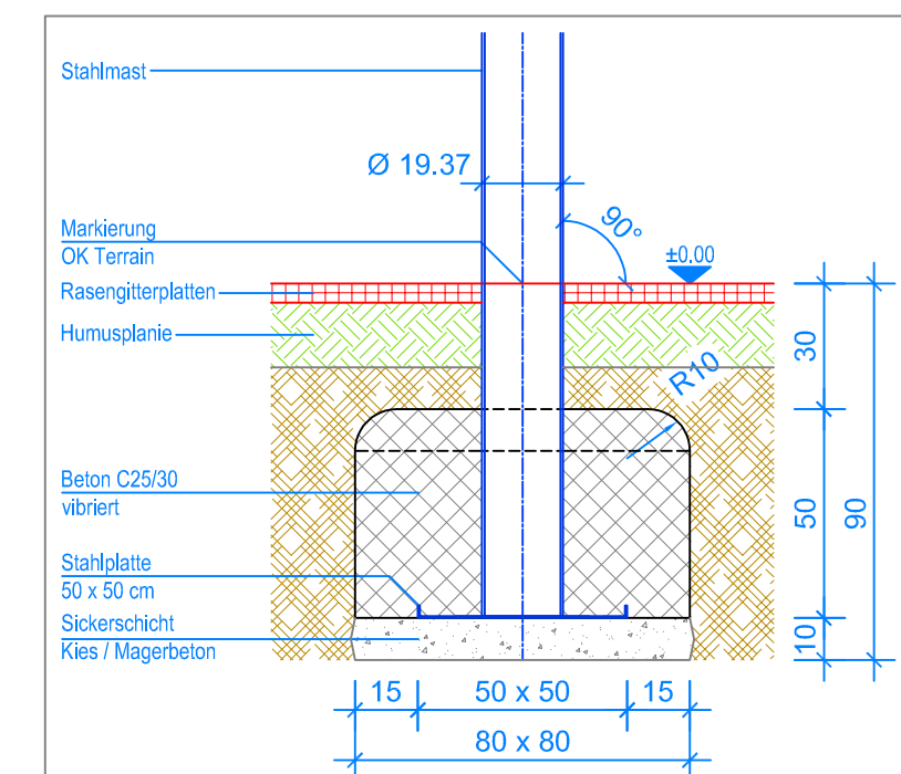
SCHNITT 1:20 FUNDAMENT STAHLMAST
