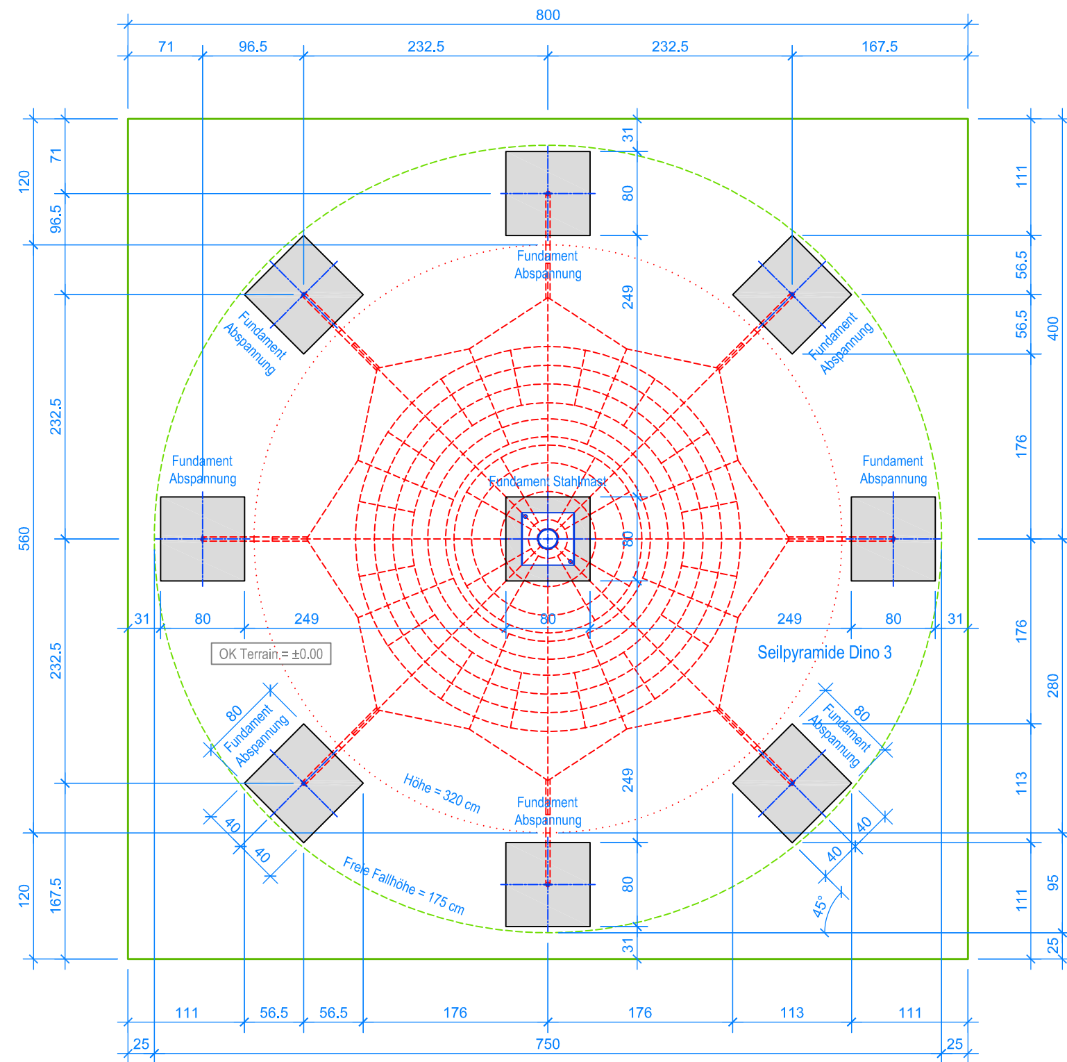
GRUNDRISS 1:50
