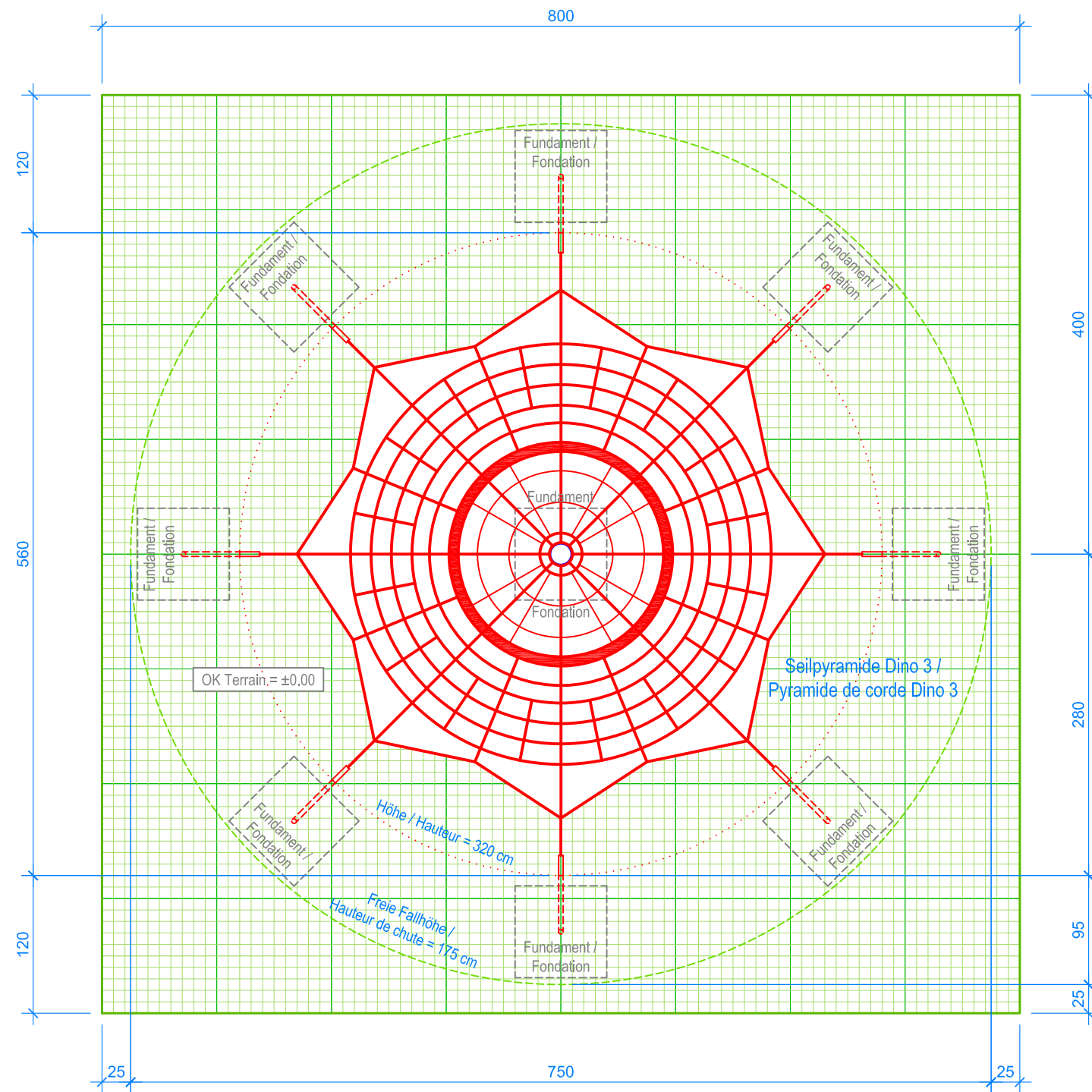
GRUNDRISS / PLAN 1:50
