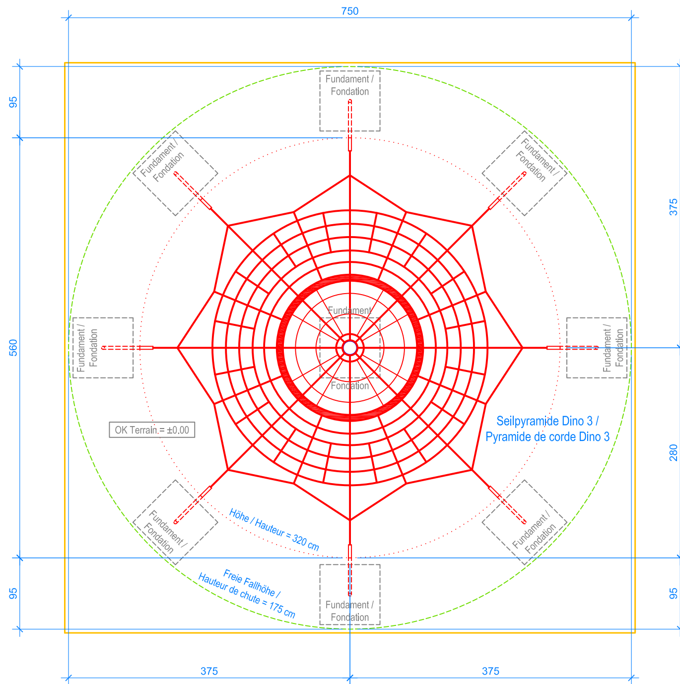
GRUNDRISS / PLAN 1:50
