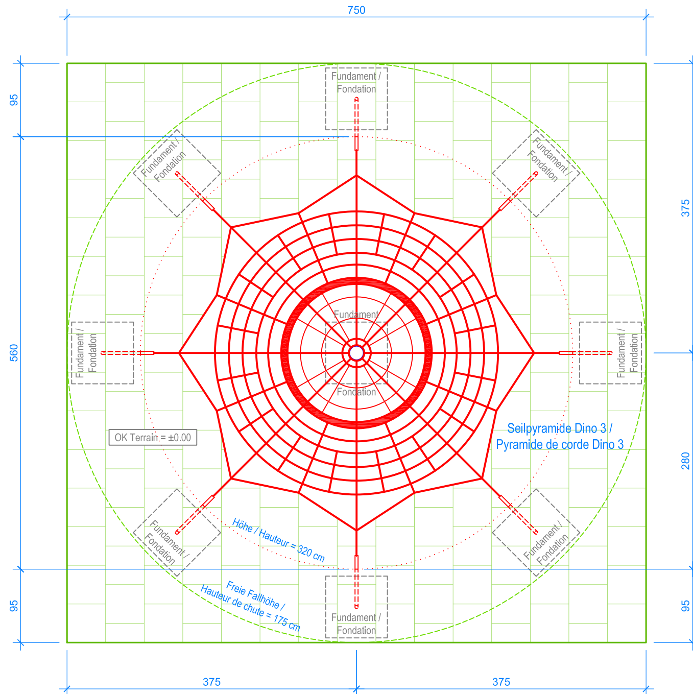
GRUNDRISS / PLAN 1:50
