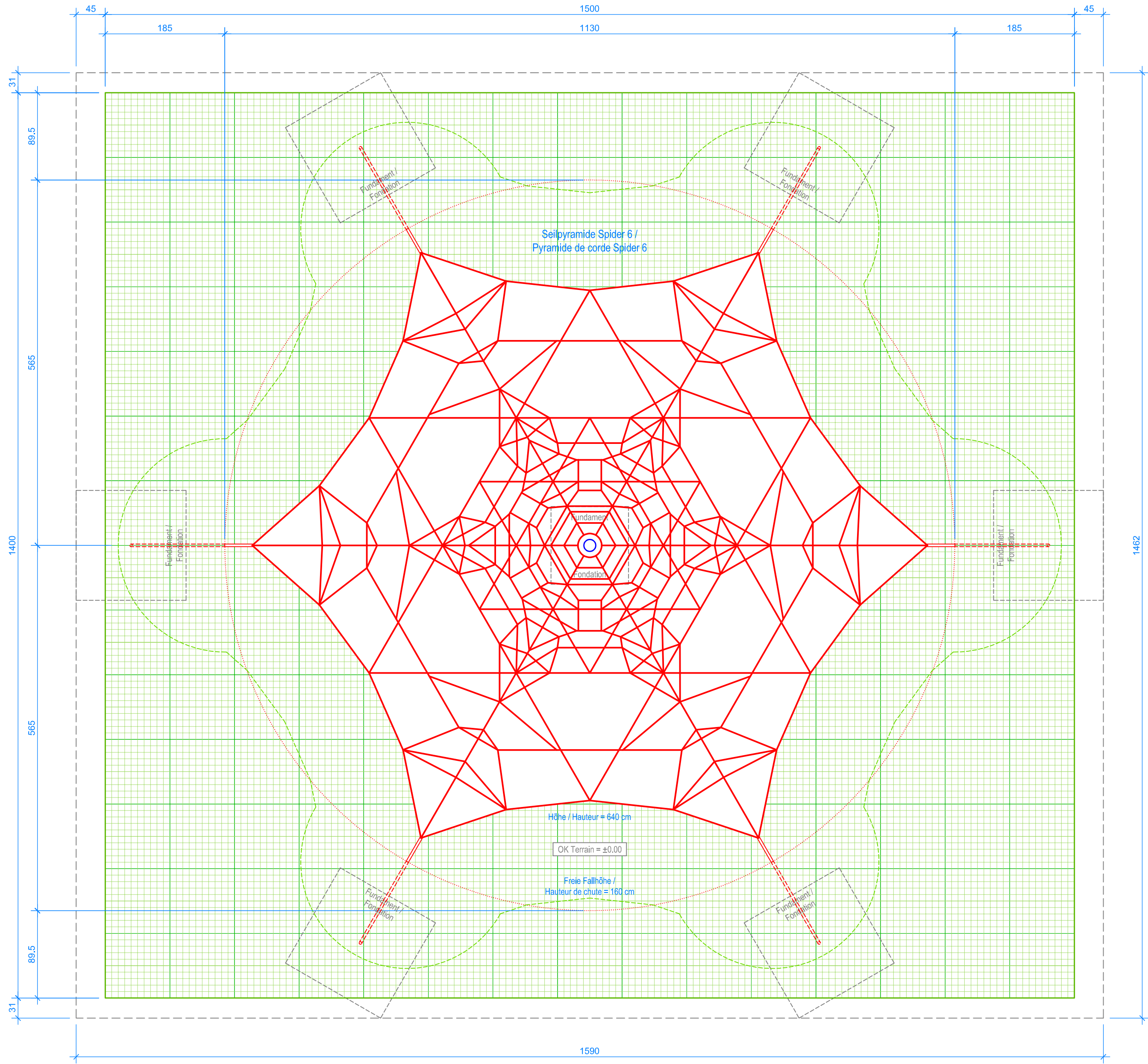
GRUNDRISS / PLAN 1:50
