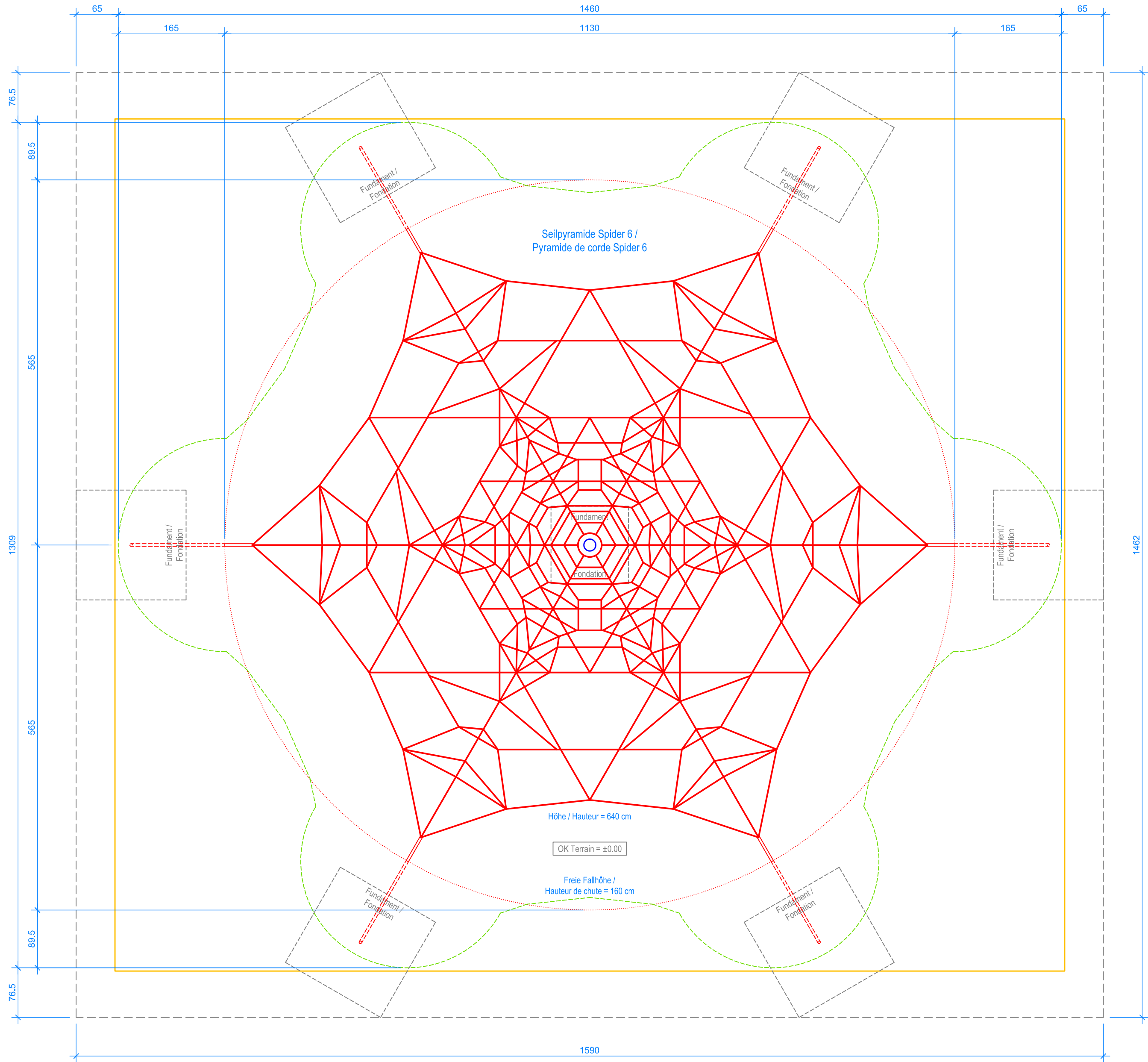
GRUNDRISS / PLAN 1:50
