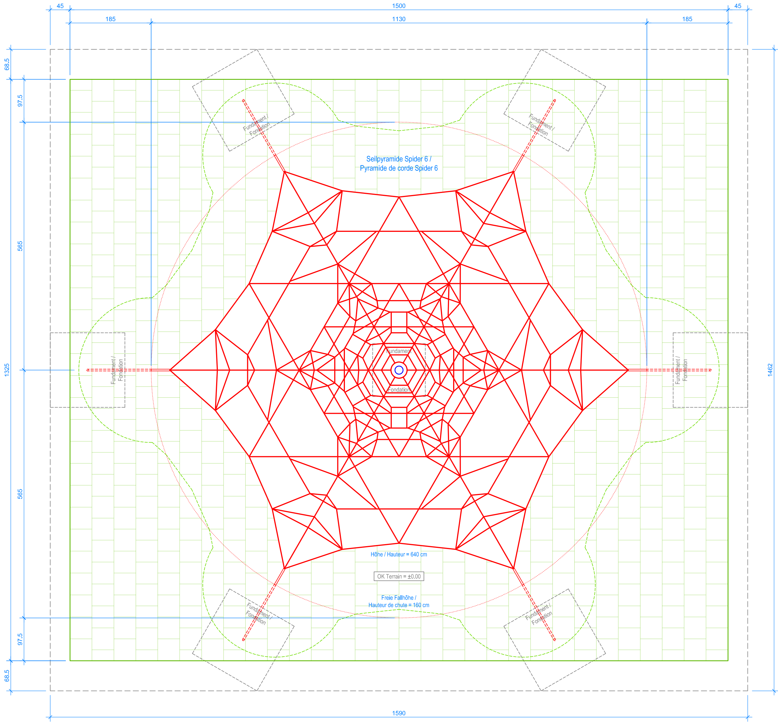
GRUNDRISS / PLAN 1:50
