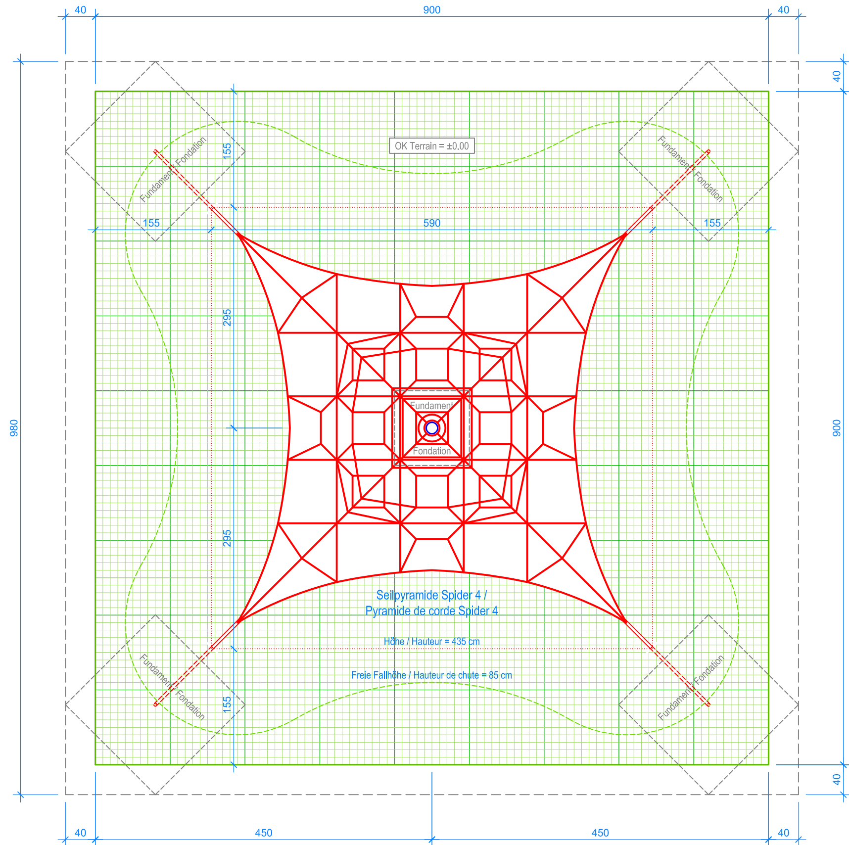
GRUNDRISS / PLAN 1:50
