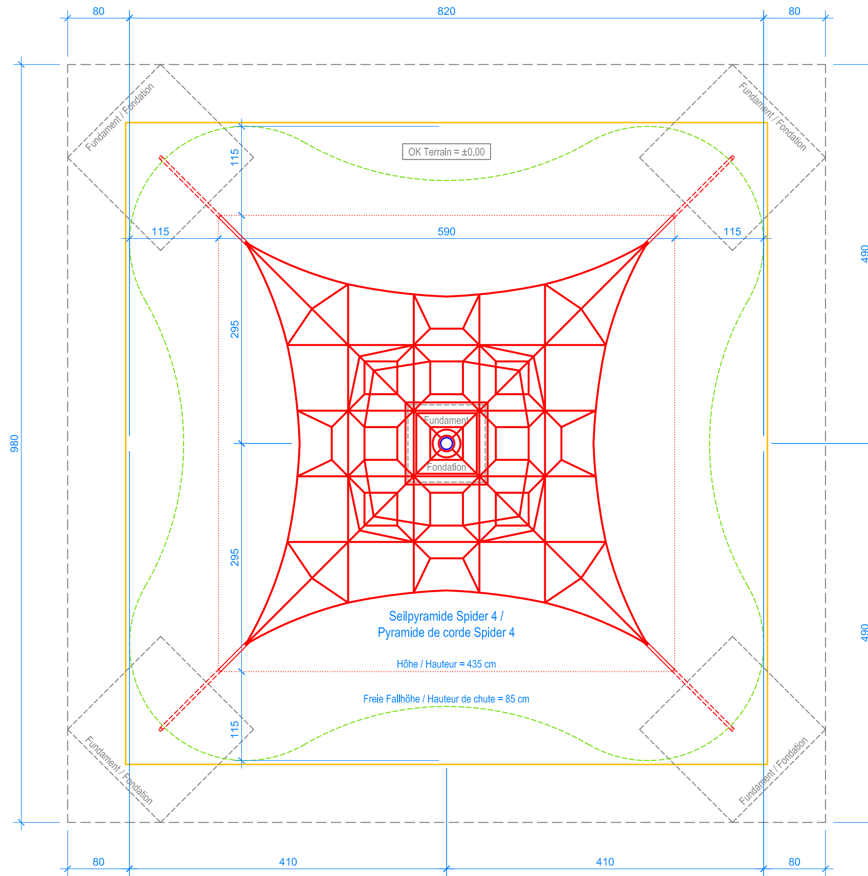
GRUNDRISS / PLAN 1:50
