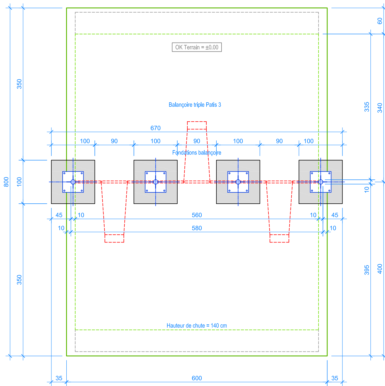
PLAN 1:50
