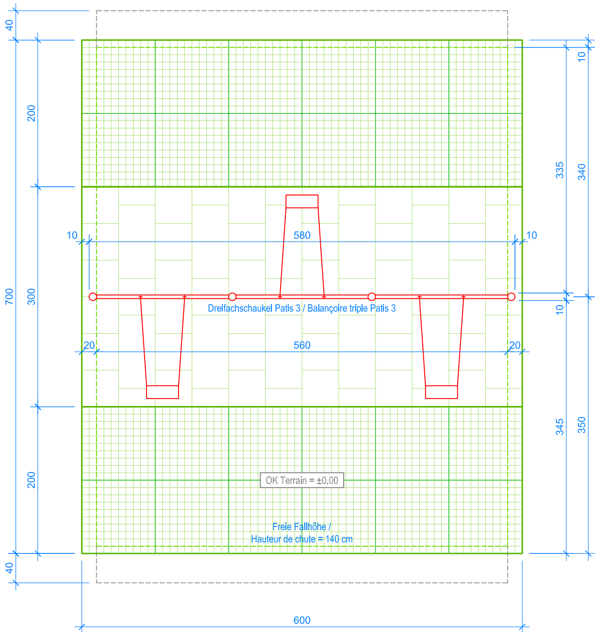
GRUNDRISS / PLAN 1:50
