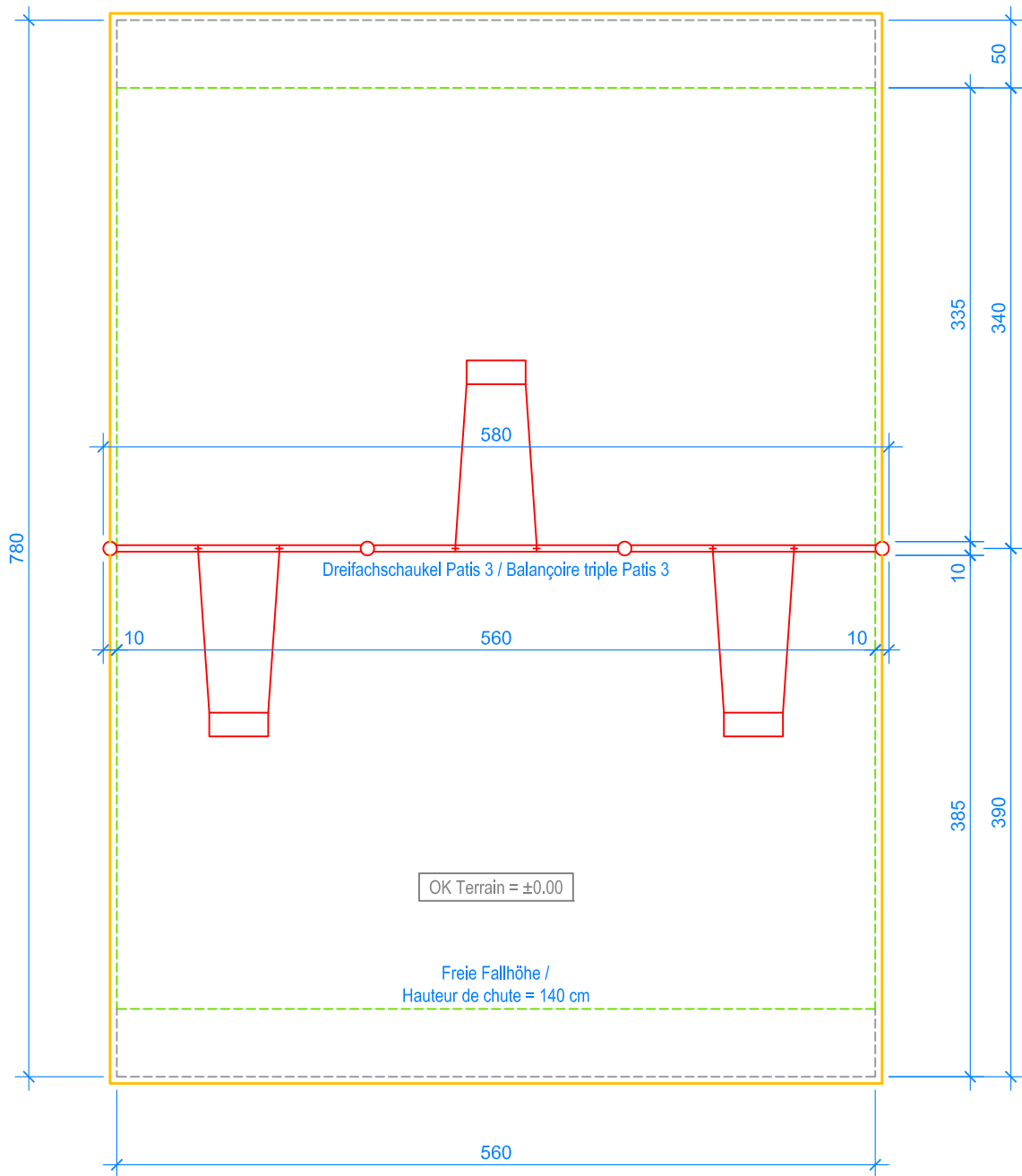
GRUNDRISS / PLAN 1:50
