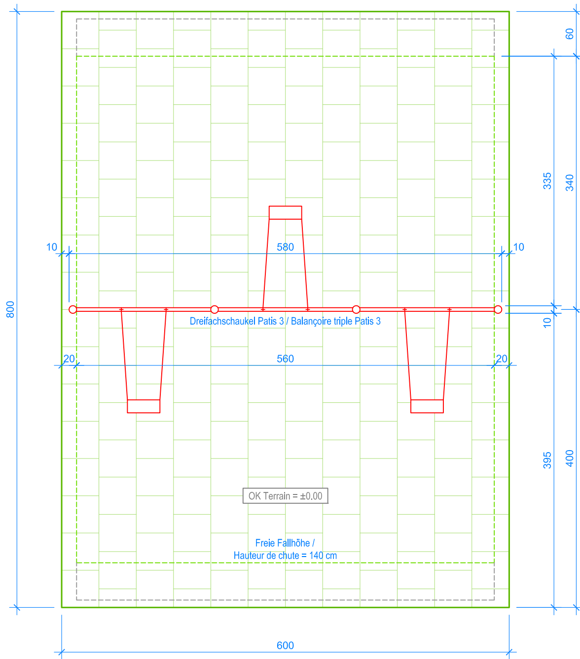
GRUNDRISS / PLAN 1:50
