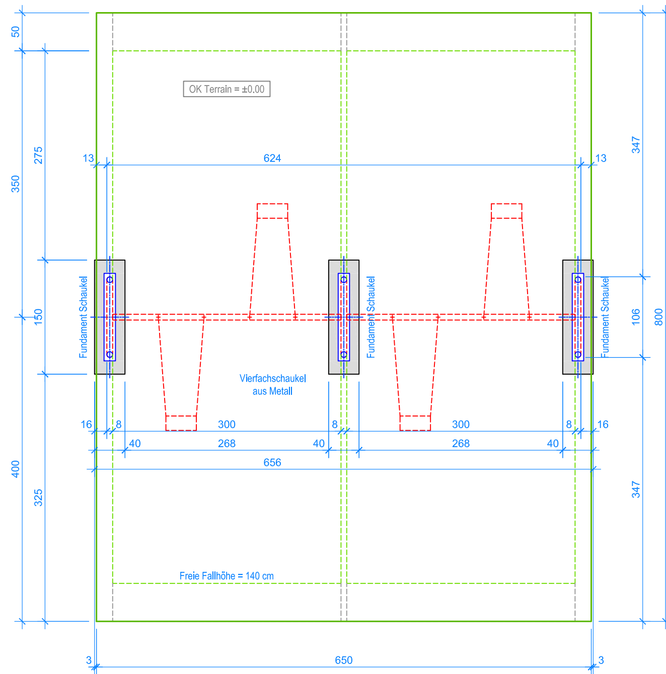
GRUNDRISS 1:50
