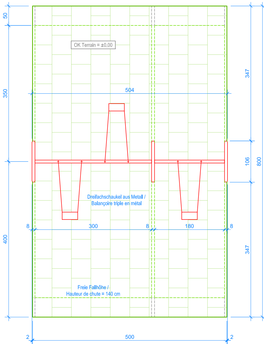
GRUNDRISS / PLAN 1:50
