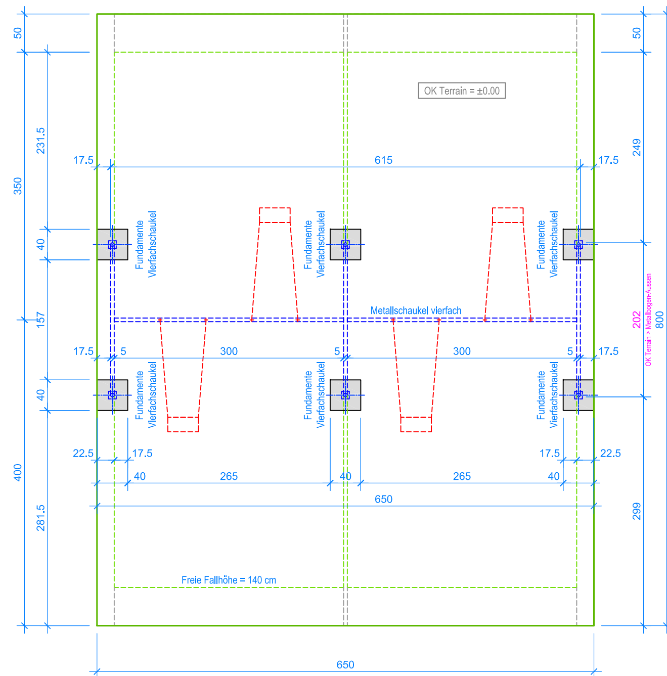
GRUNDRISS 1:50
