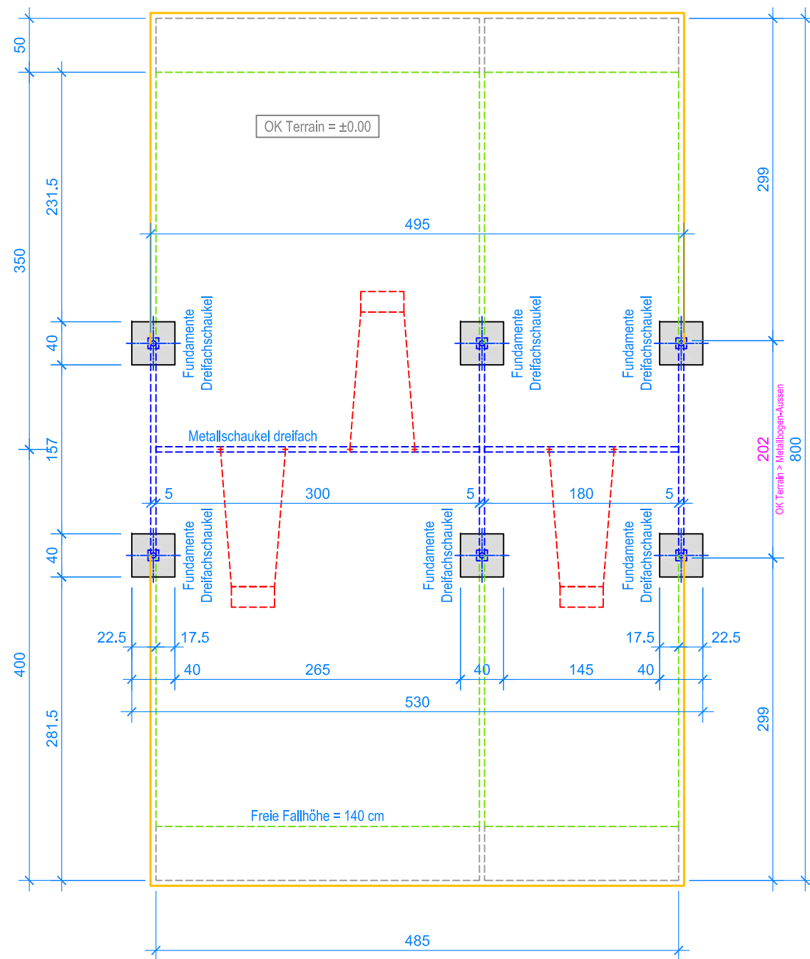
GRUNDRISS 1:50
