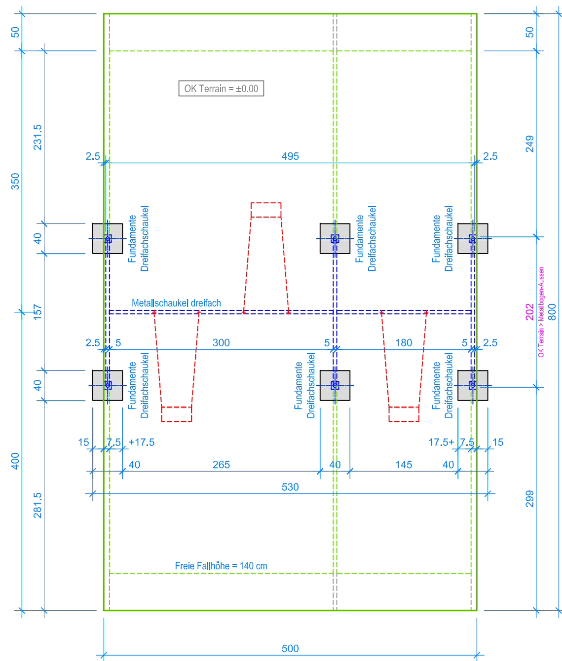
GRUNDRISS 1:50
