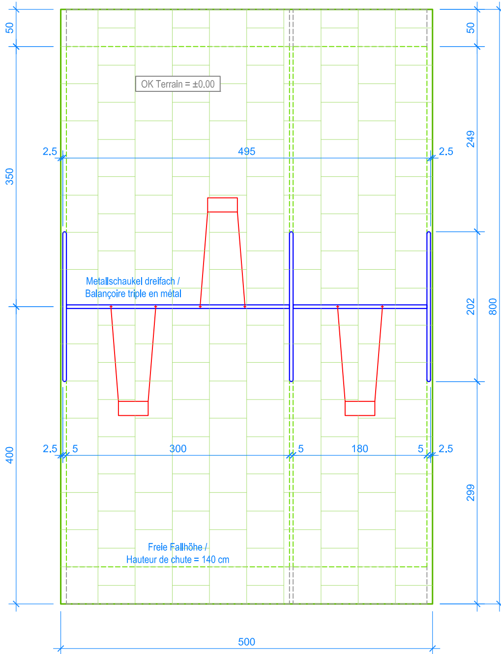
GRUNDRISS / PLAN 1:50
