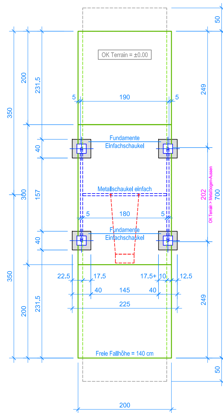
GRUNDRISS 1:50
