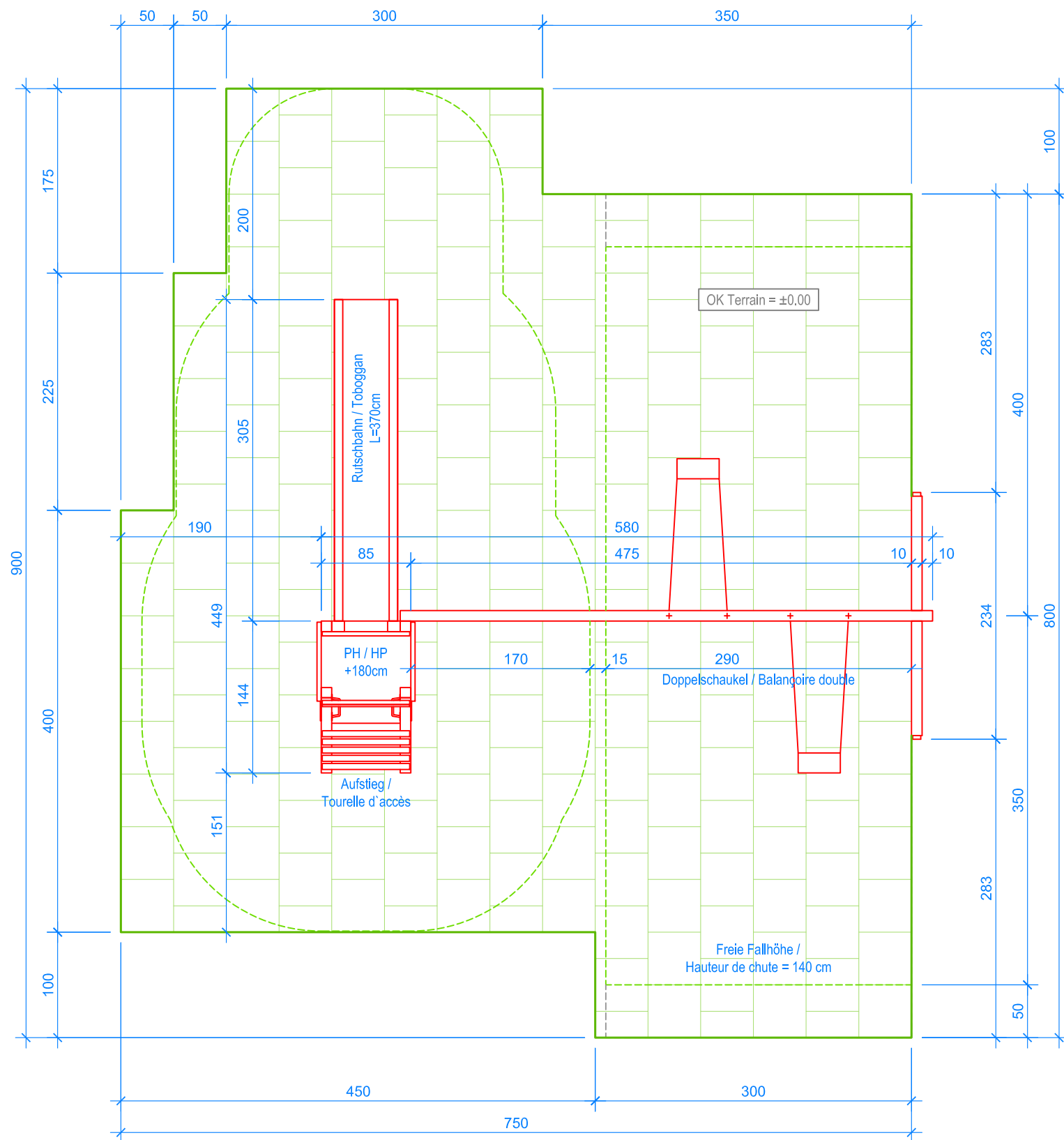
GRUNDRISS / PLAN 1:50
