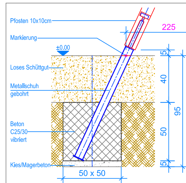
SCHNITT 1:20 FUNDAMENT DOPPELSCHAUKEL
