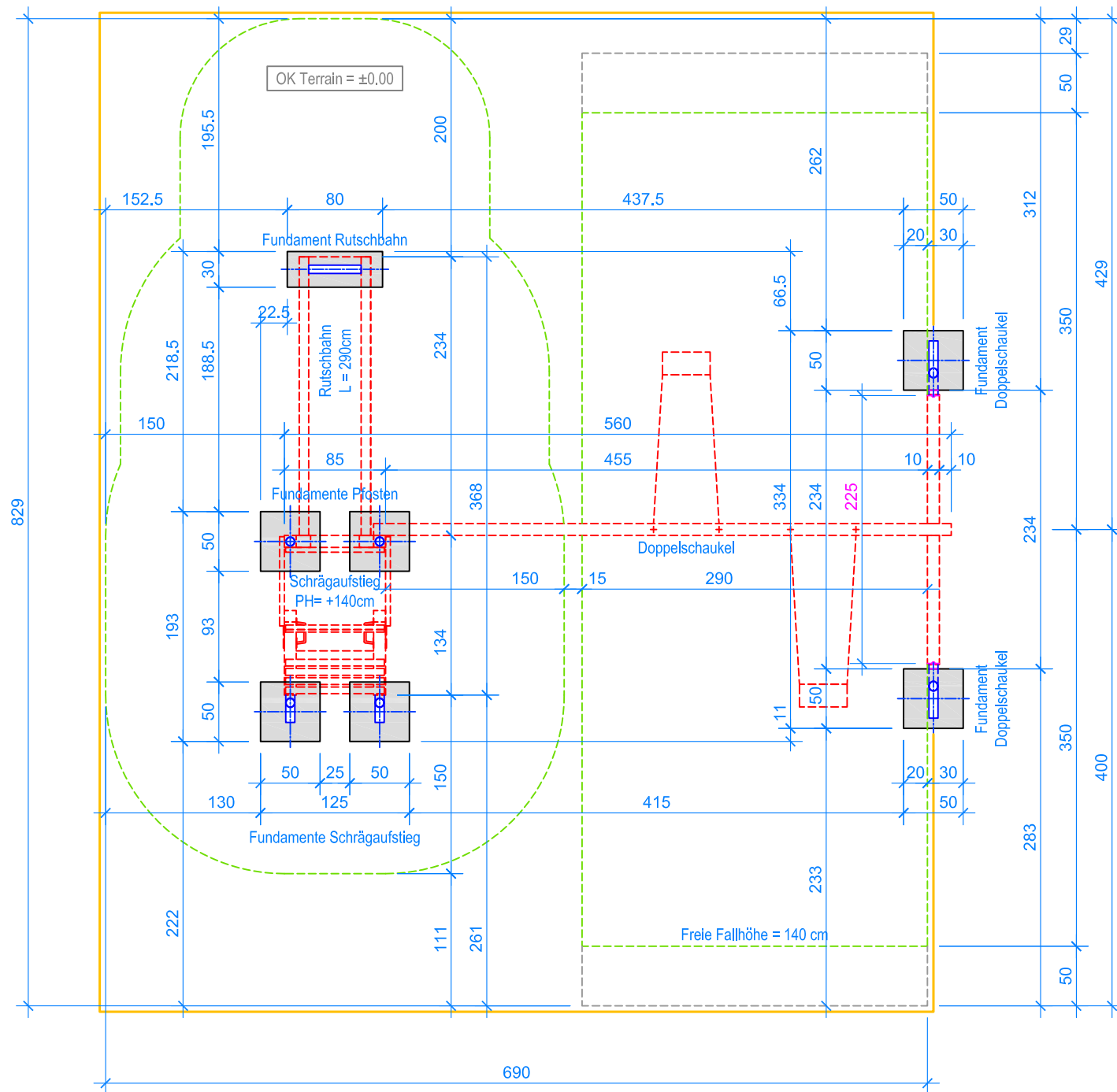
GRUNDRISS 1:50
