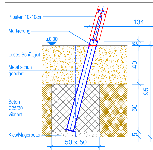
SCHNITT 1:20 FUNDAMENT SCHRÄGAUFSTIEG
