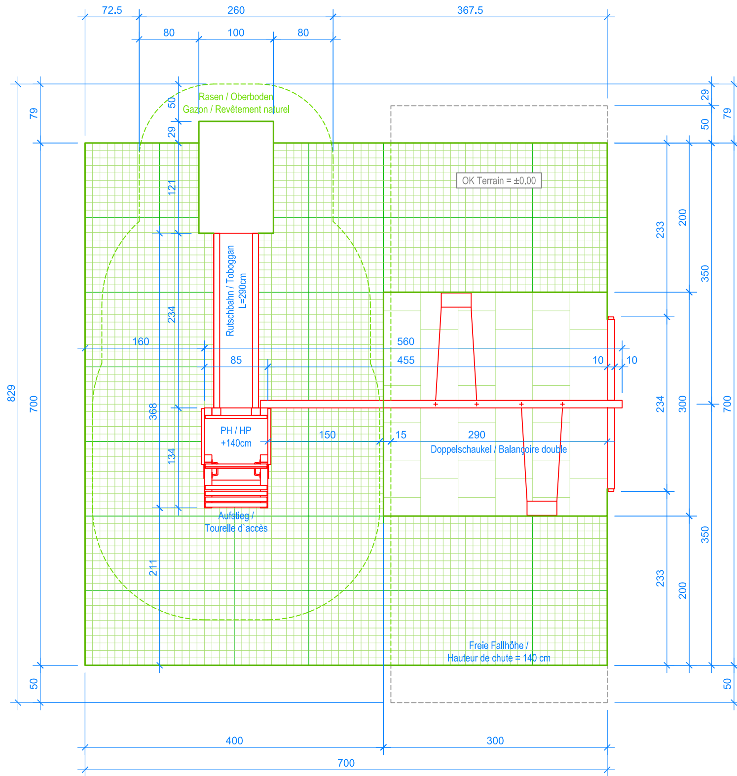
GRUNDRISS / PLAN 1:50
