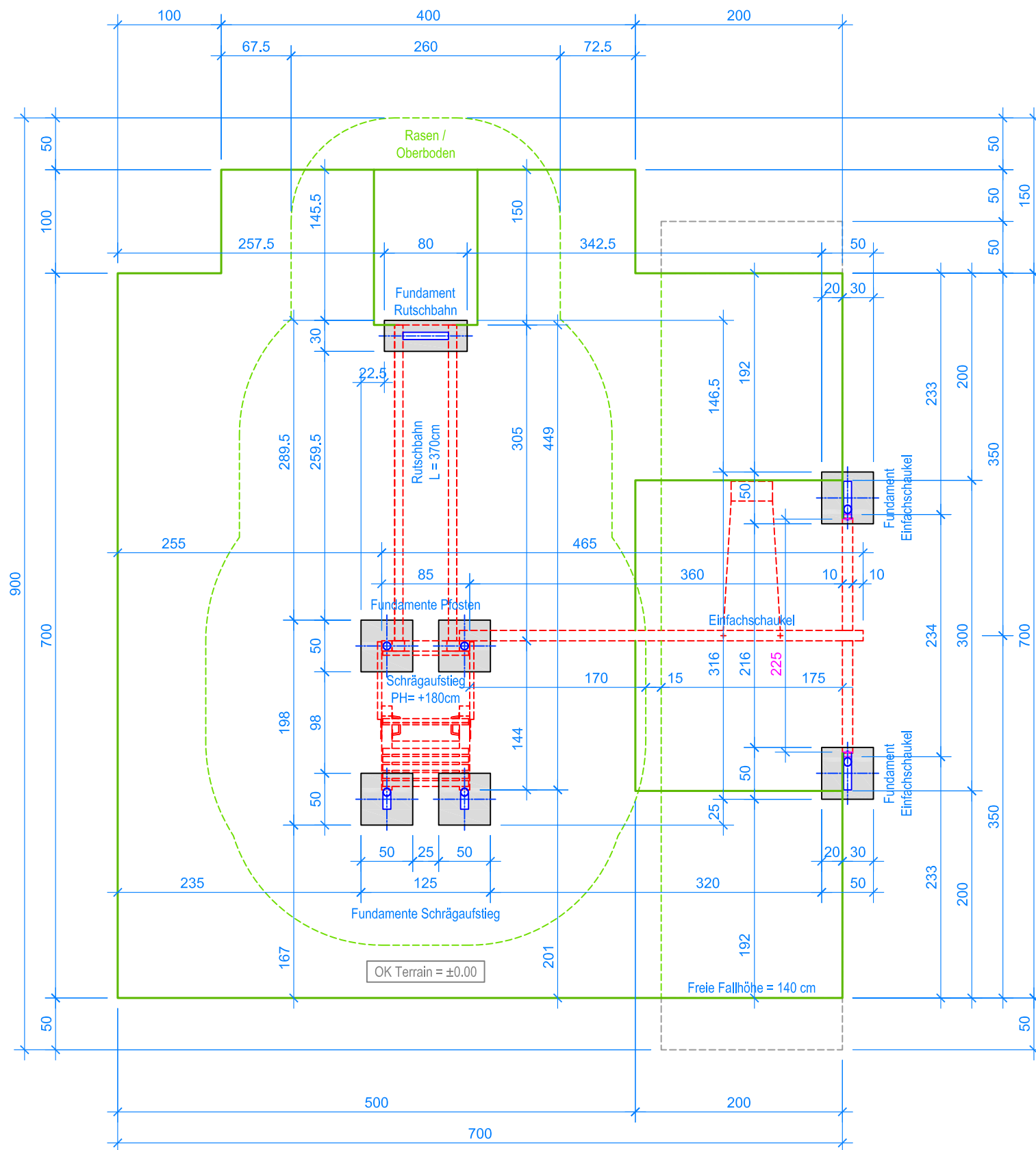
GRUNDRISS 1:50
