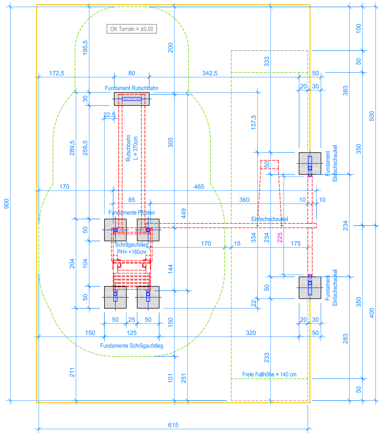
GRUNDRISS 1:50
