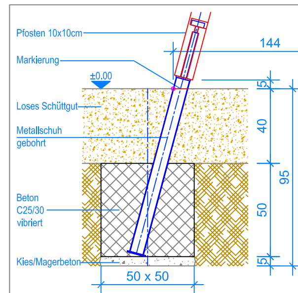
SCHNITT 1:20 FUNDAMENT SCHRÄGAUFSTIEG
