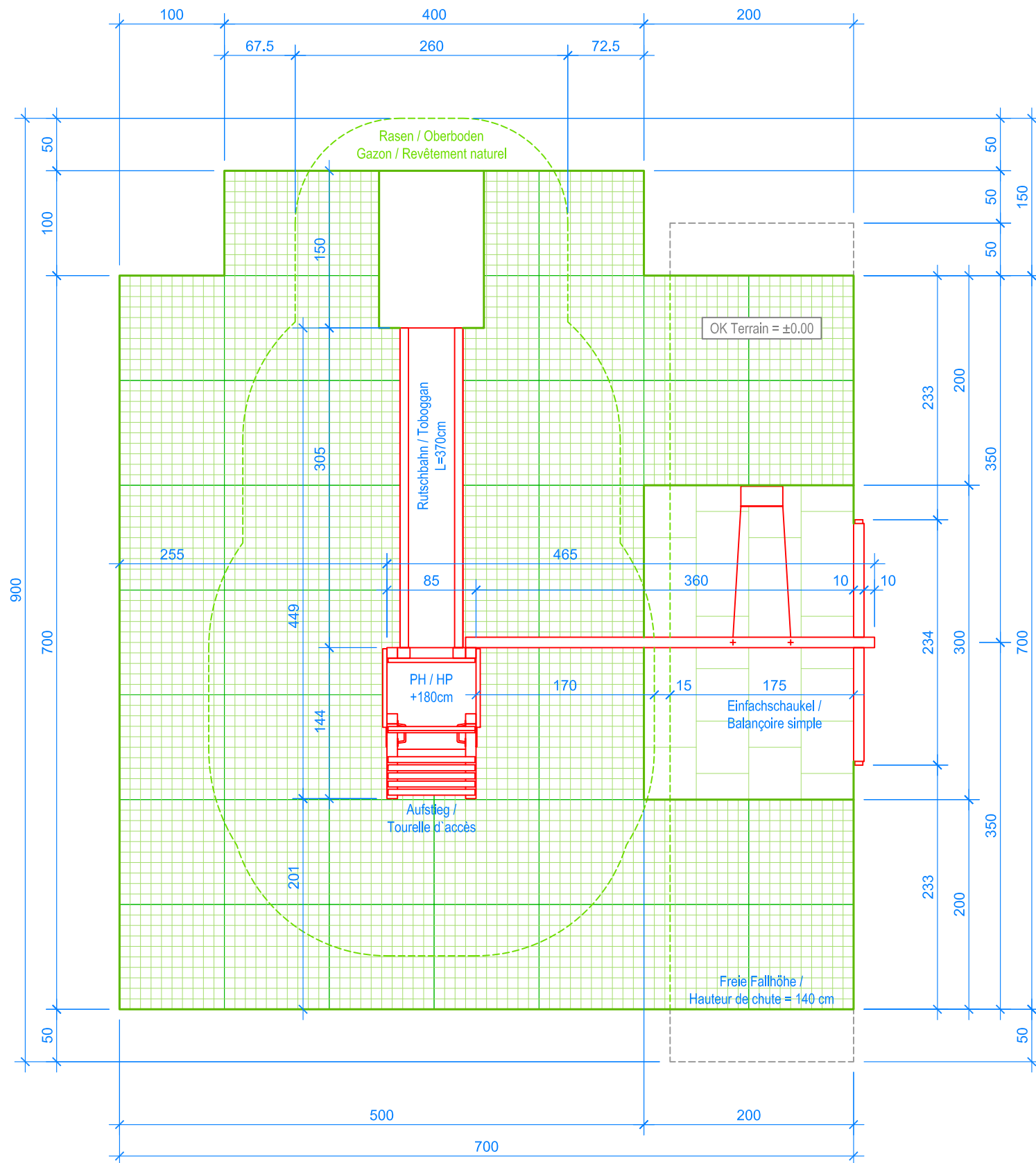
GRUNDRISS / PLAN 1:50
