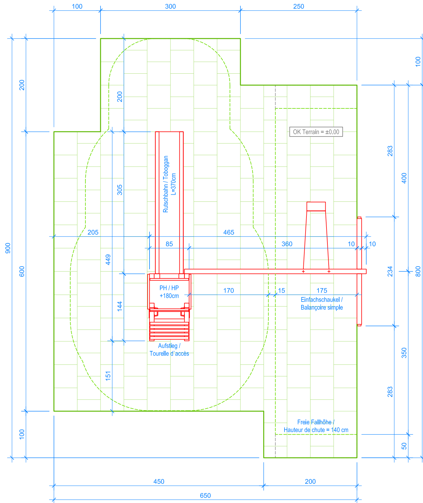
GRUNDRISS / PLAN 1:50
