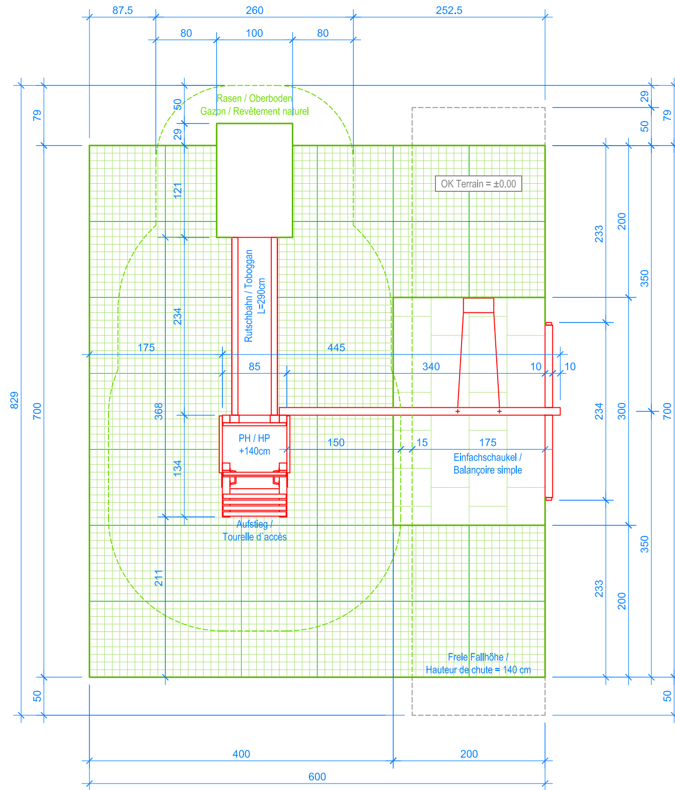
GRUNDRISS / PLAN 1:50
