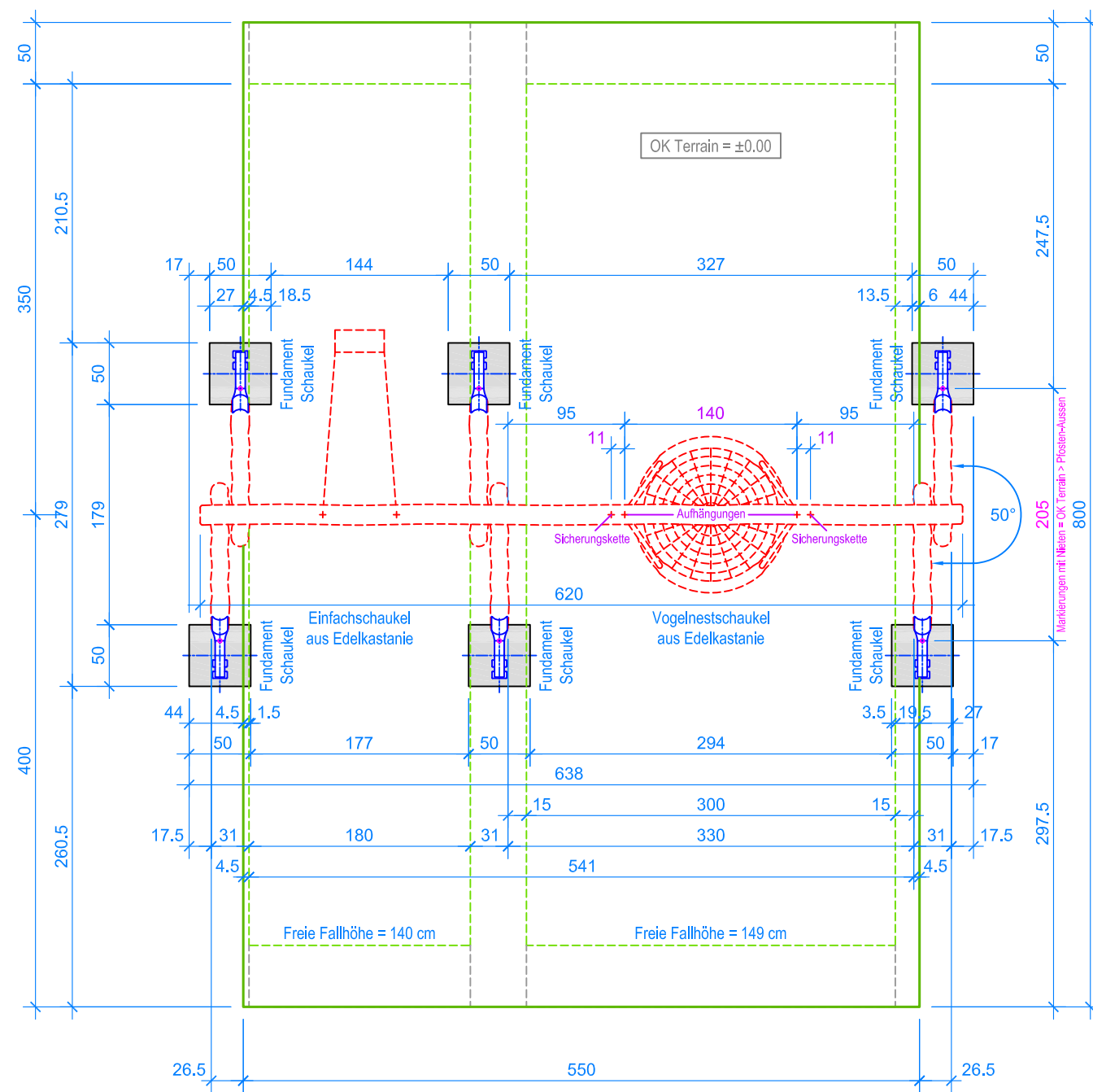
GRUNDRISS 1:50
