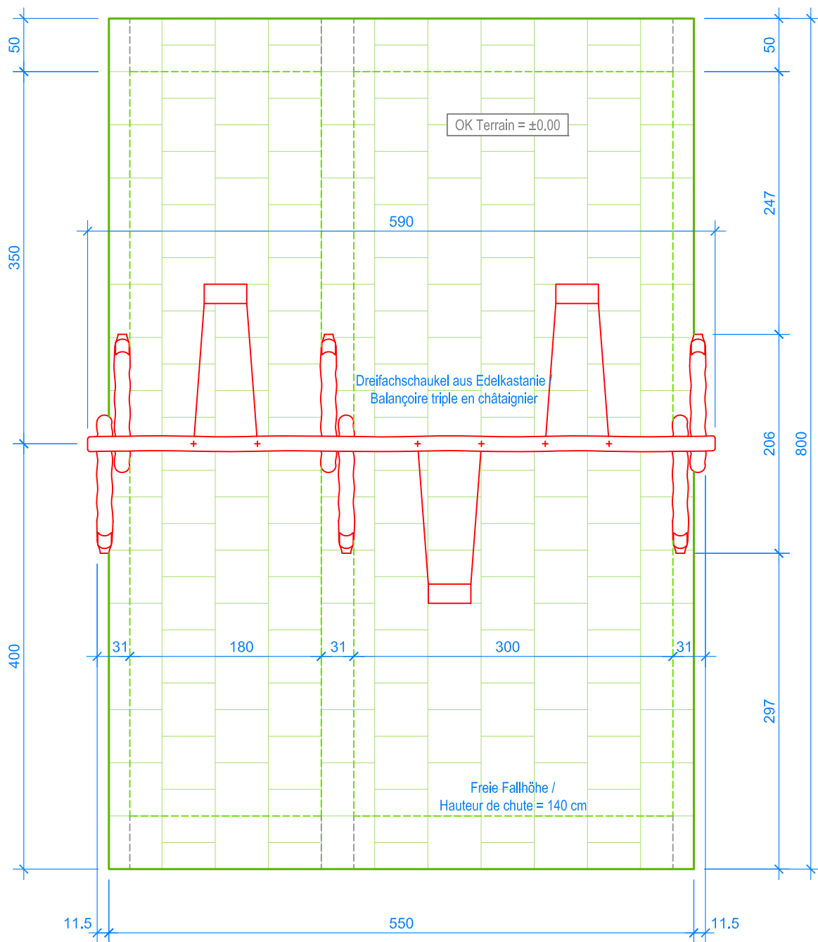
GRUNDRISS / PLAN 1:50
