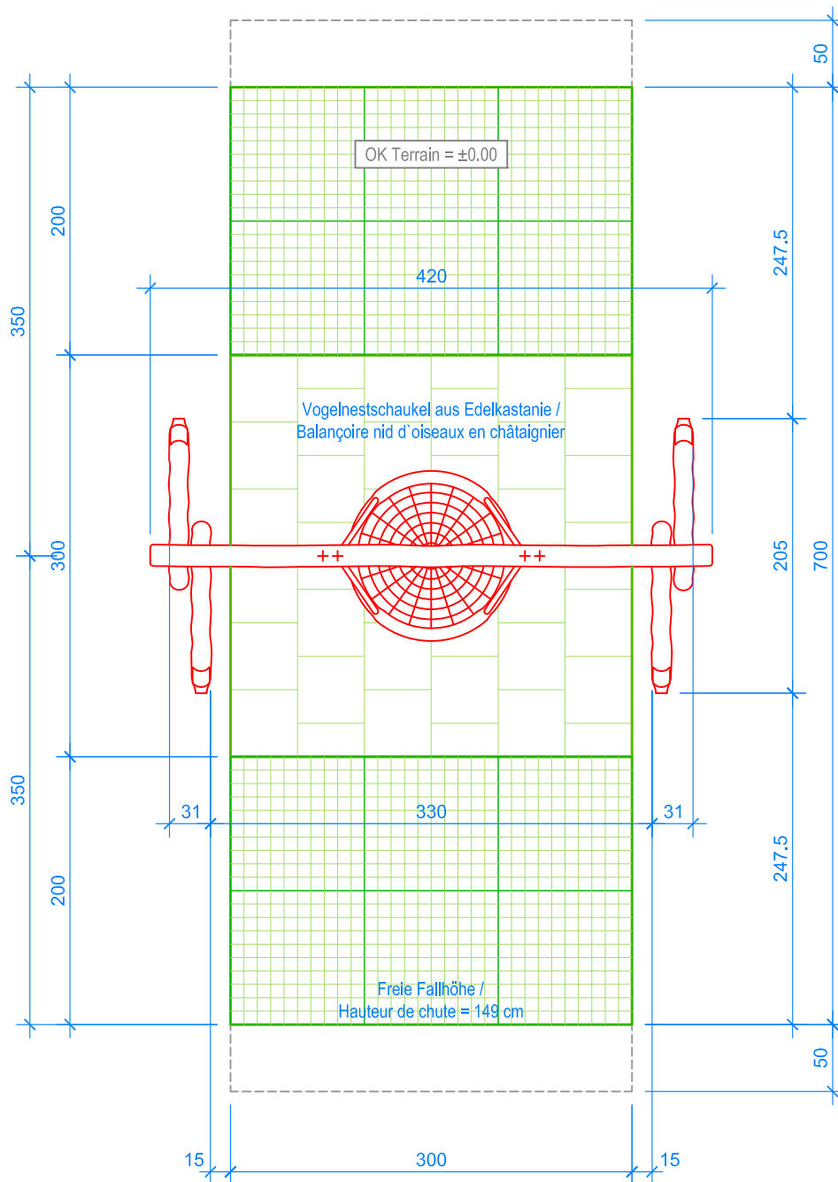
GRUNDRISS / PLAN 1:50
