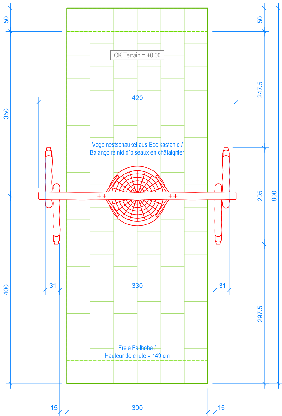
GRUNDRISS / PLAN 1:50
