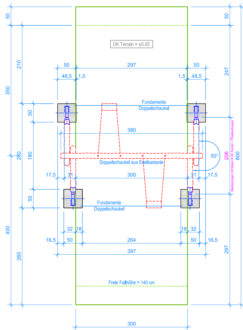
GRUNDRISS 1:50
