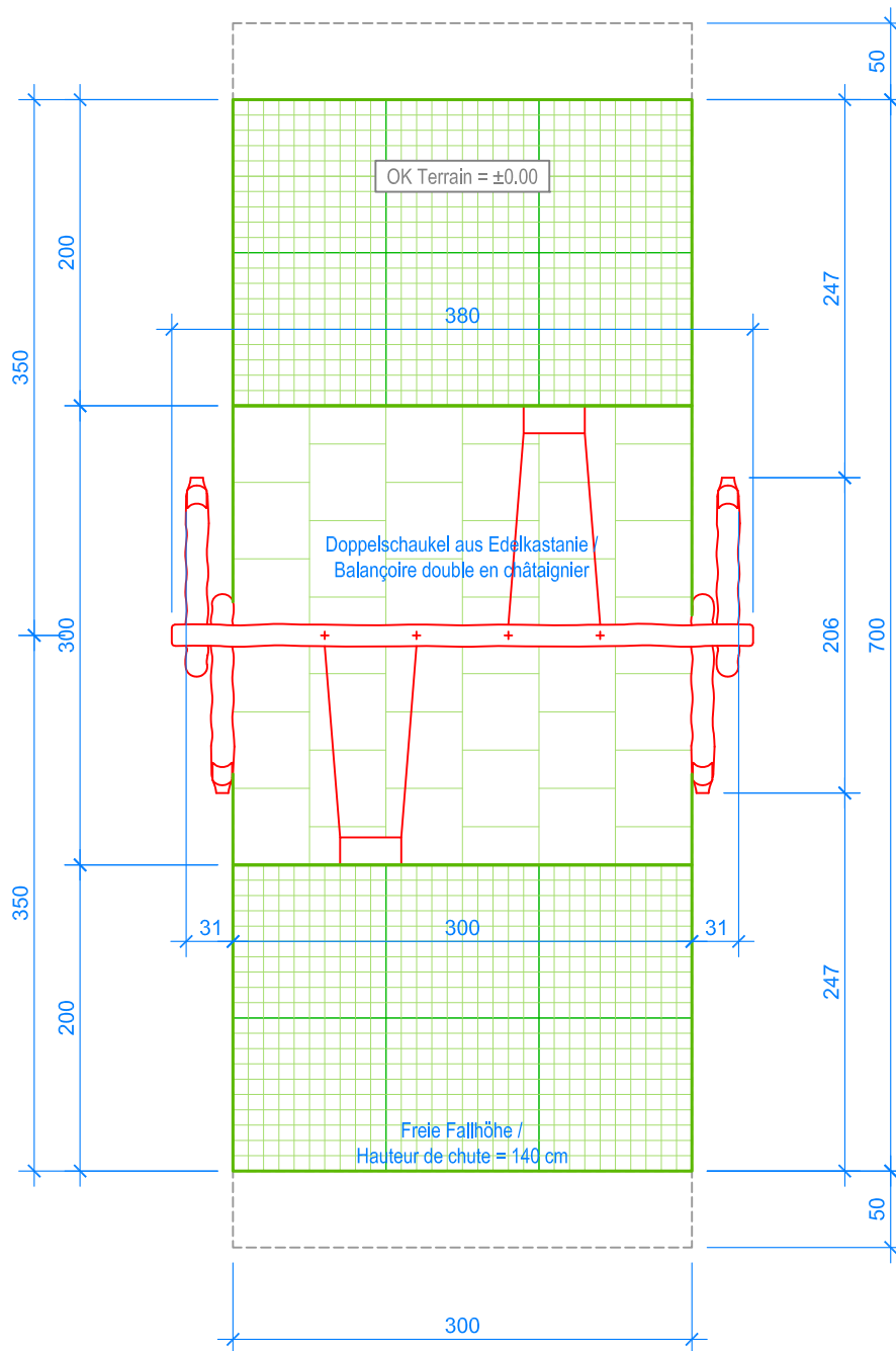
GRUNDRISS / PLAN 1:50
