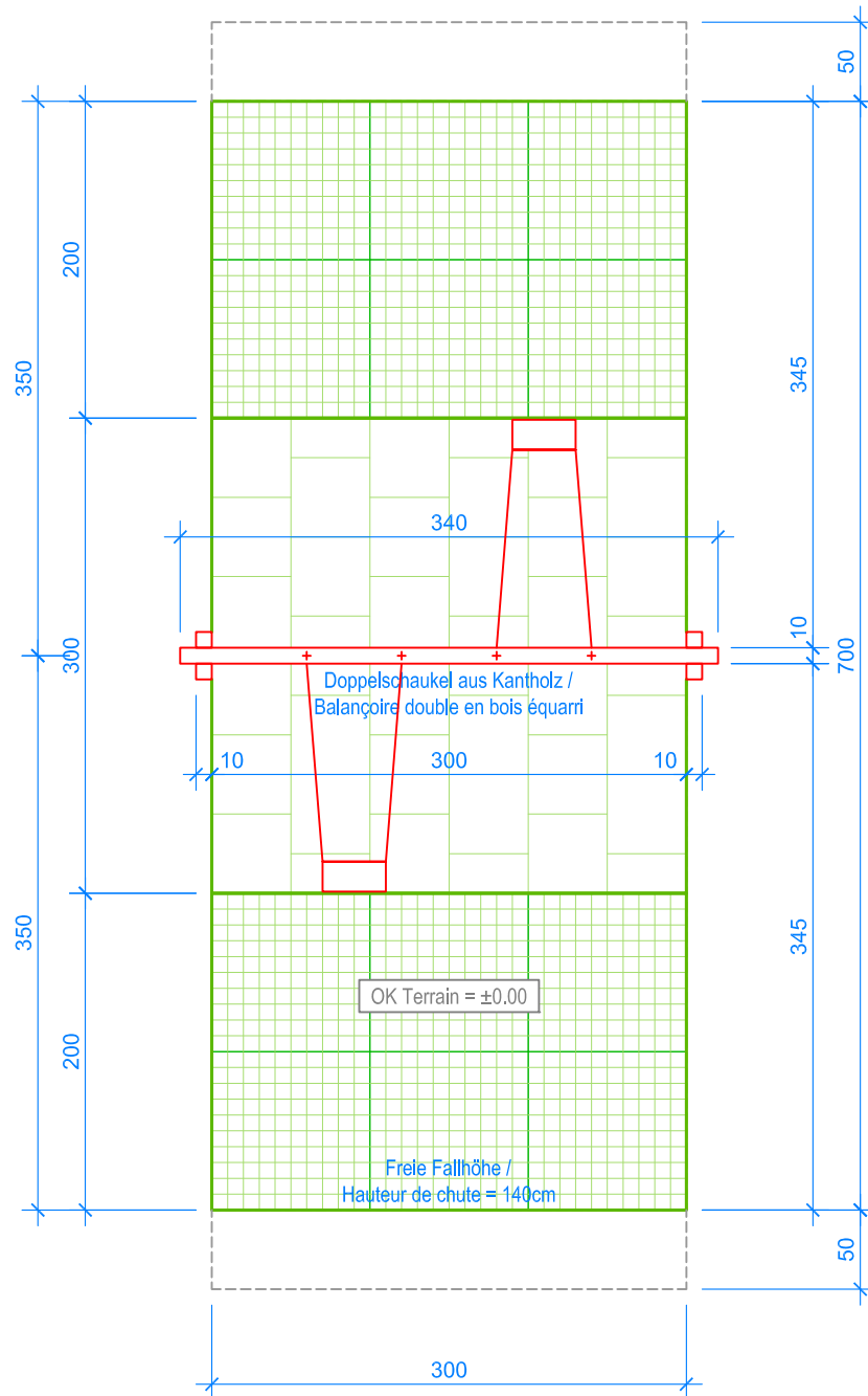
GRUNDRISS / PLAN 1:50
