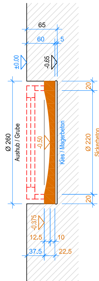
SCHNITT B-B 1:50
