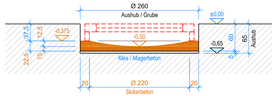
SCHNITT A-A 1:50
