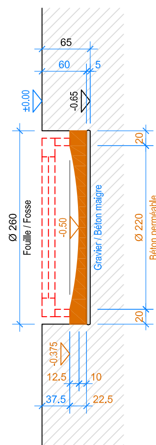
COUPE B-B 1:50
