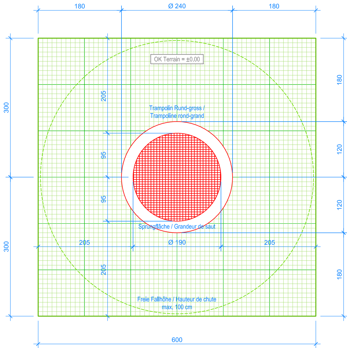
GRUNDRISS / PLAN 1:50
