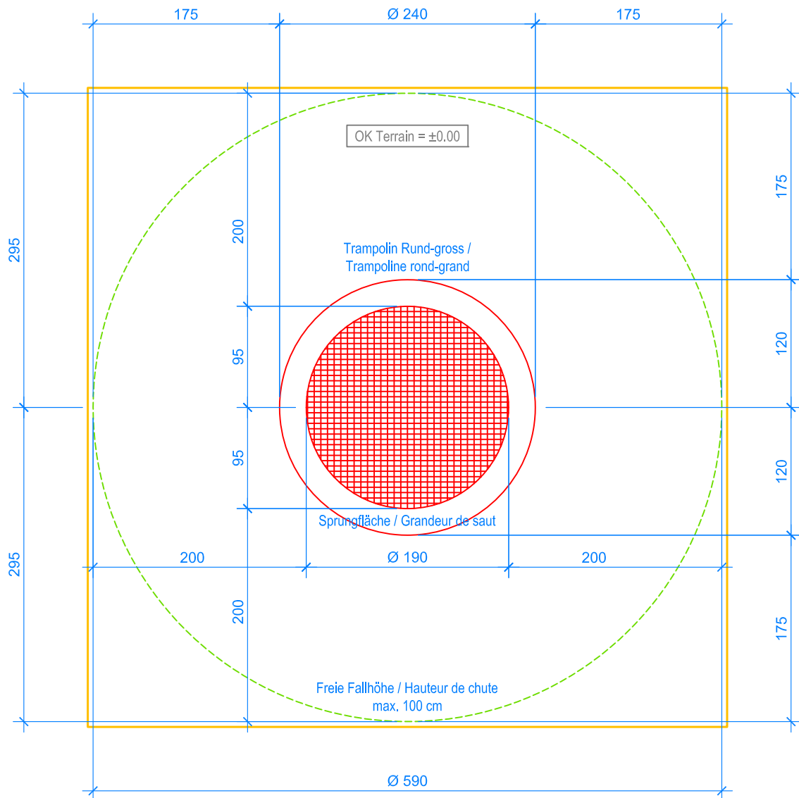
GRUNDRISS / PLAN 1:50
