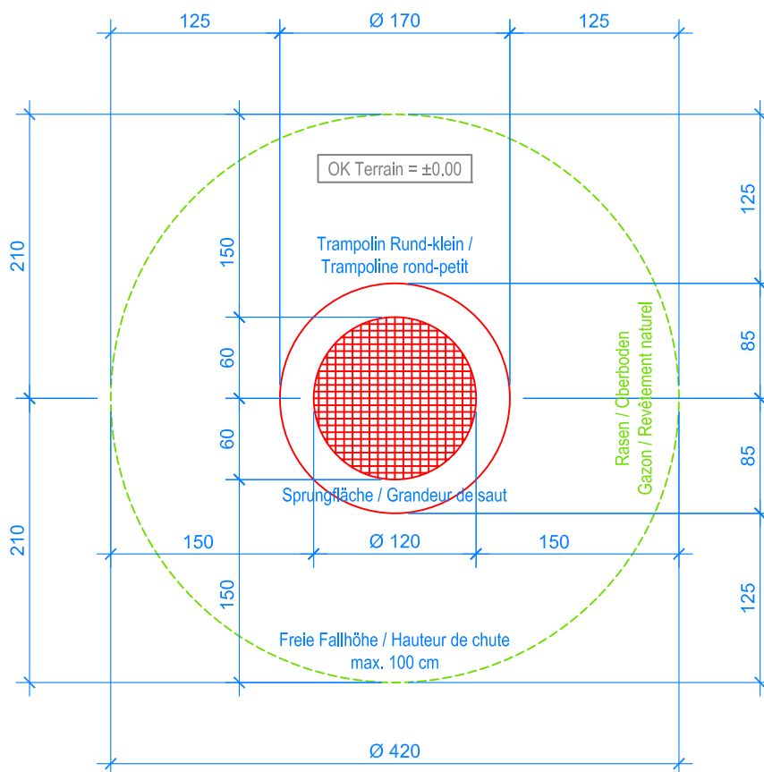
GRUNDRISS / PLAN 1:50
