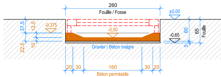
COUPE A-A 1:50
