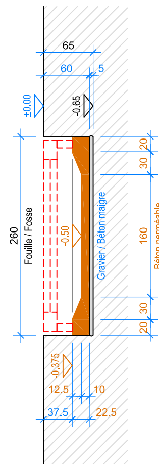
COUPE B-B 1:50
