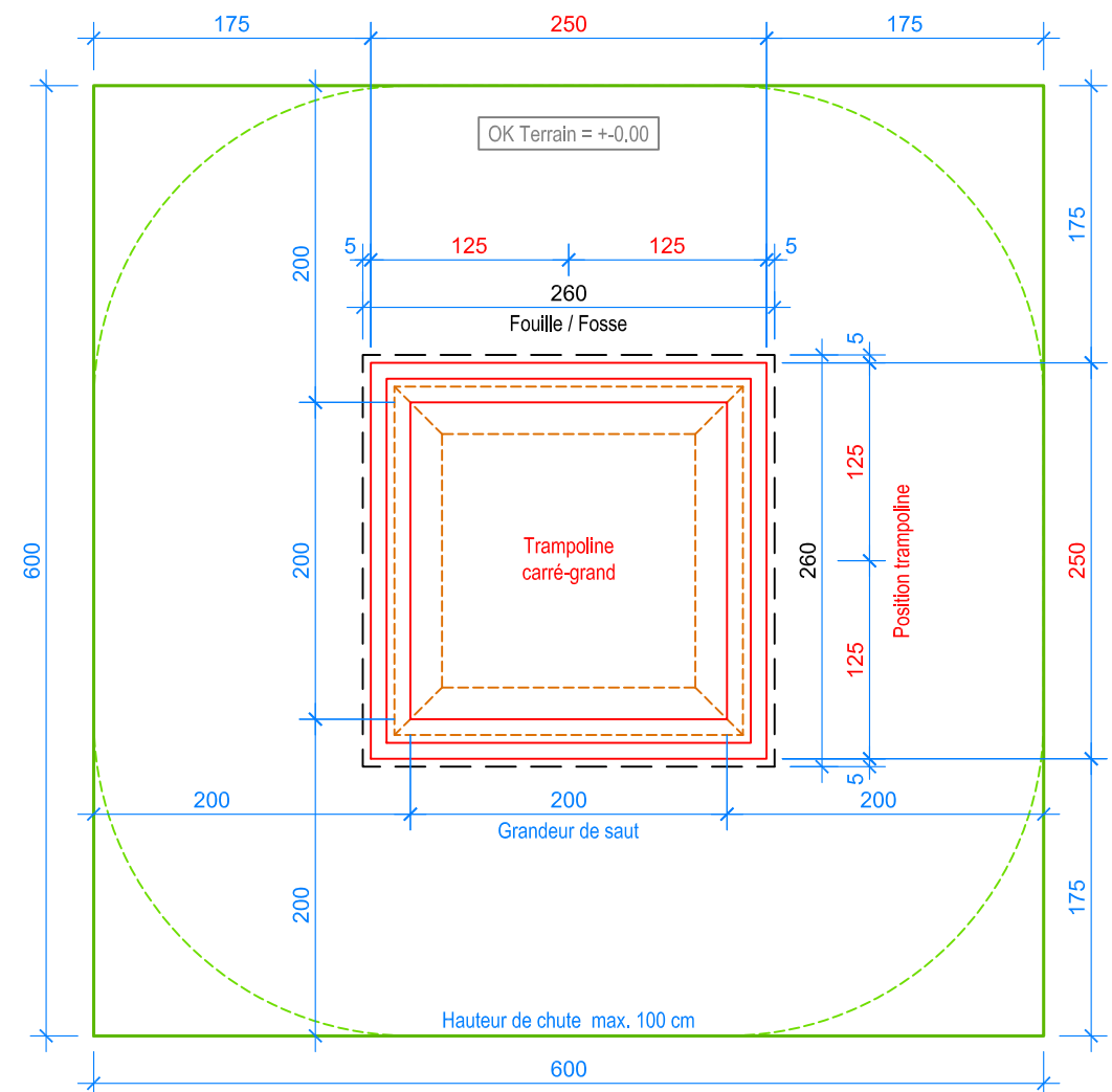
PLAN 1:50
