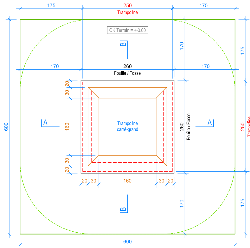
PLAN 1:50
