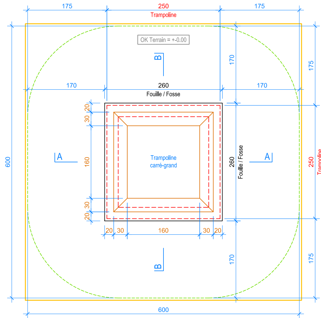
PLAN 1:50
