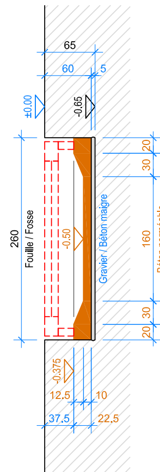
COUPE B-B 1:50
